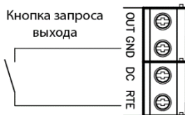
Рис.5. Подключение кнопки запроса прохода
