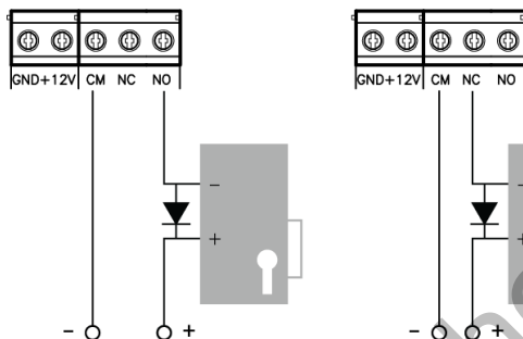
Рис.7. Подключение замков
