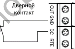
Рис.6. Подключение дверного контакта
