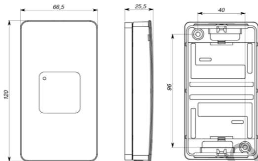
Рис 2. Габаритные размеры
