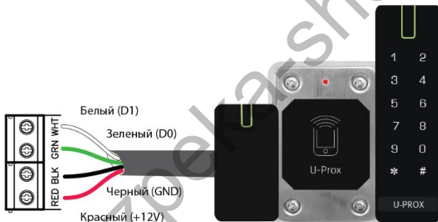
Рис. 4. Подключение считывателя
