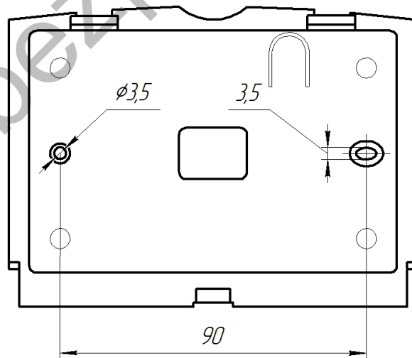
Рисунок Г.2 – Установчі розміри клавіатури
