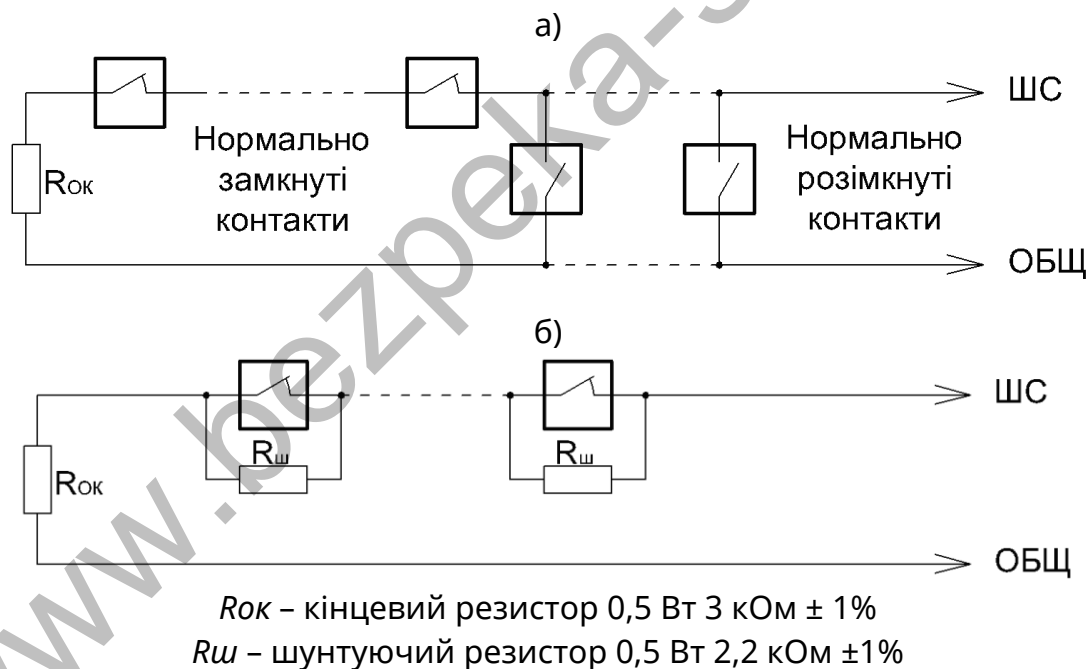
Рисунок 2 – Схеми підключення:
