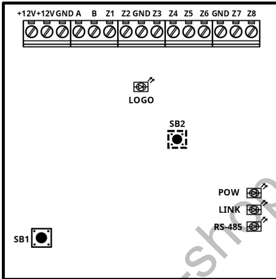
Рисунок 2 - Зовнішній вигляд плати модуля
