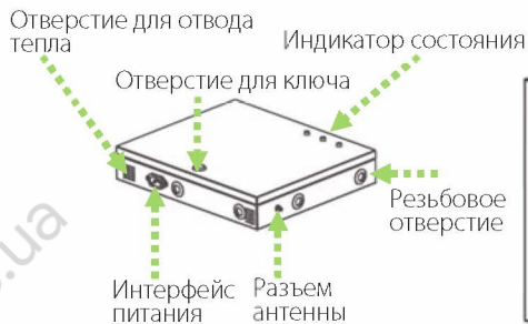
Внешний вид панели
