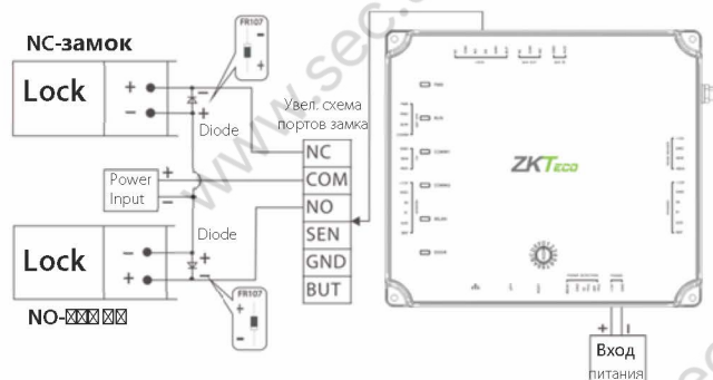
Схема подключения в сухом режиме замка с внешним источником питания (рекомендуется)
