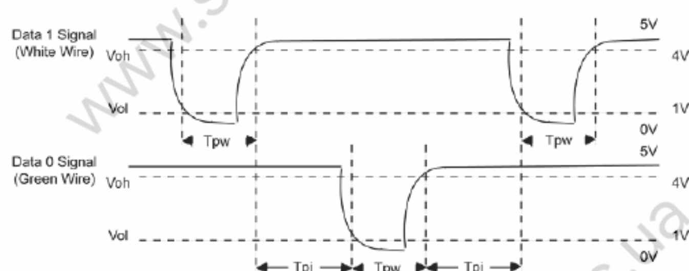
Рис.1: Діаграма послідовності
