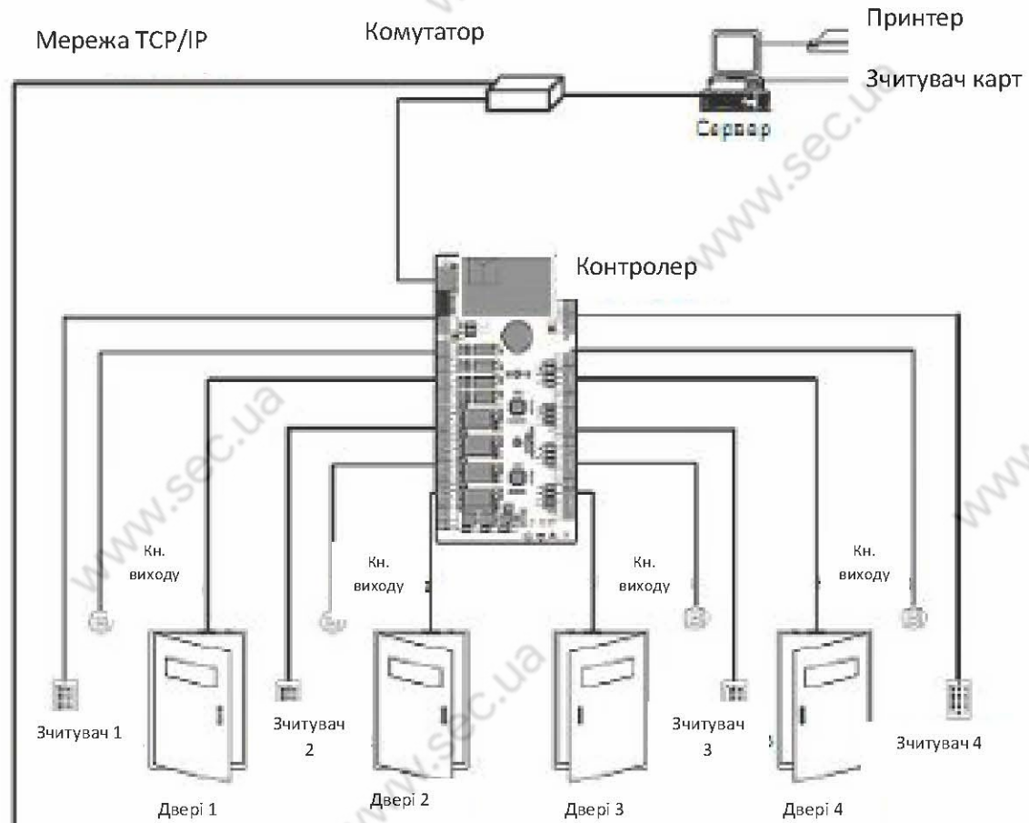
Управління 4-ма односторонніми дверима
