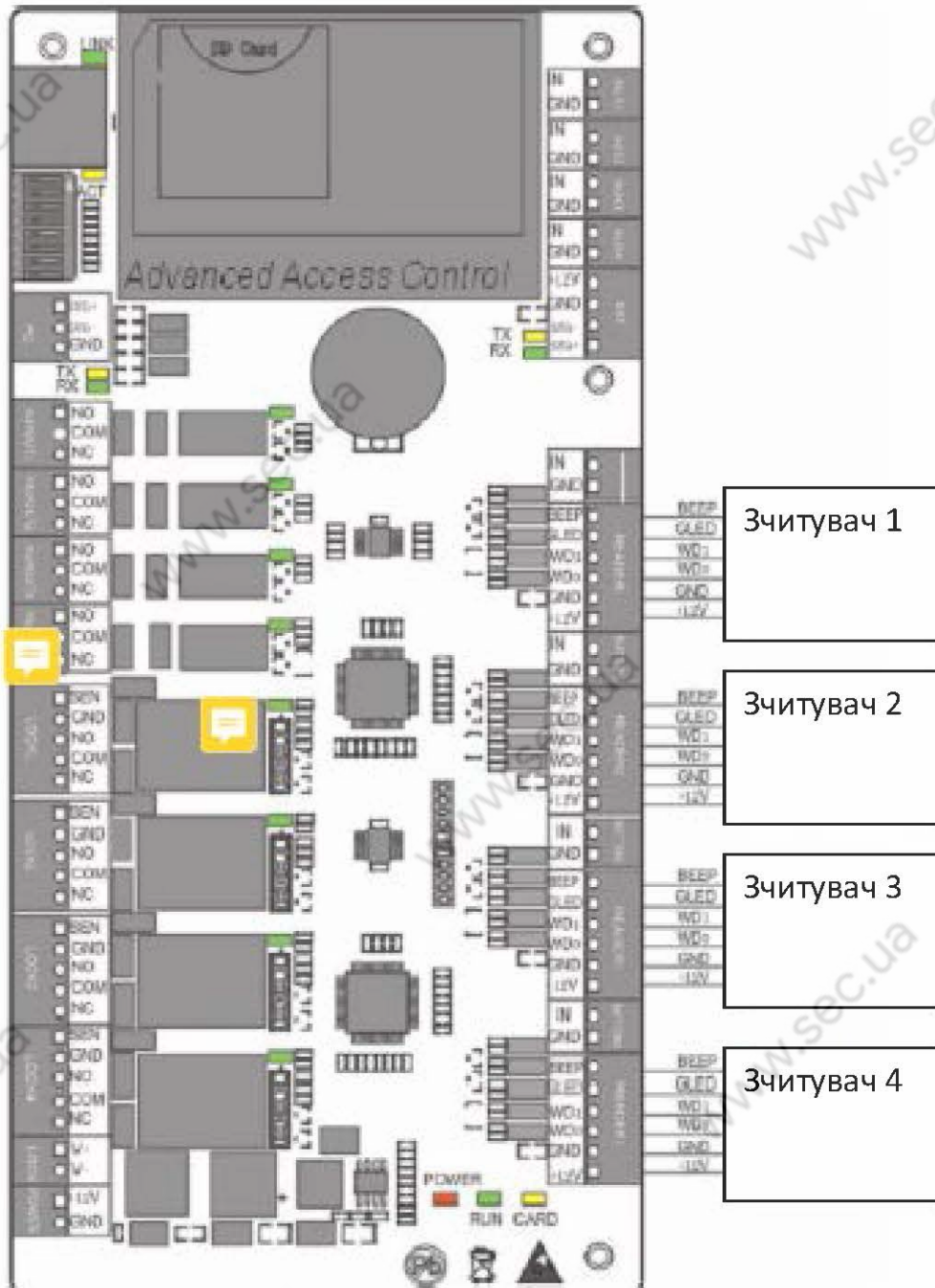
Підключення зчитувачів до контролера С3-400
