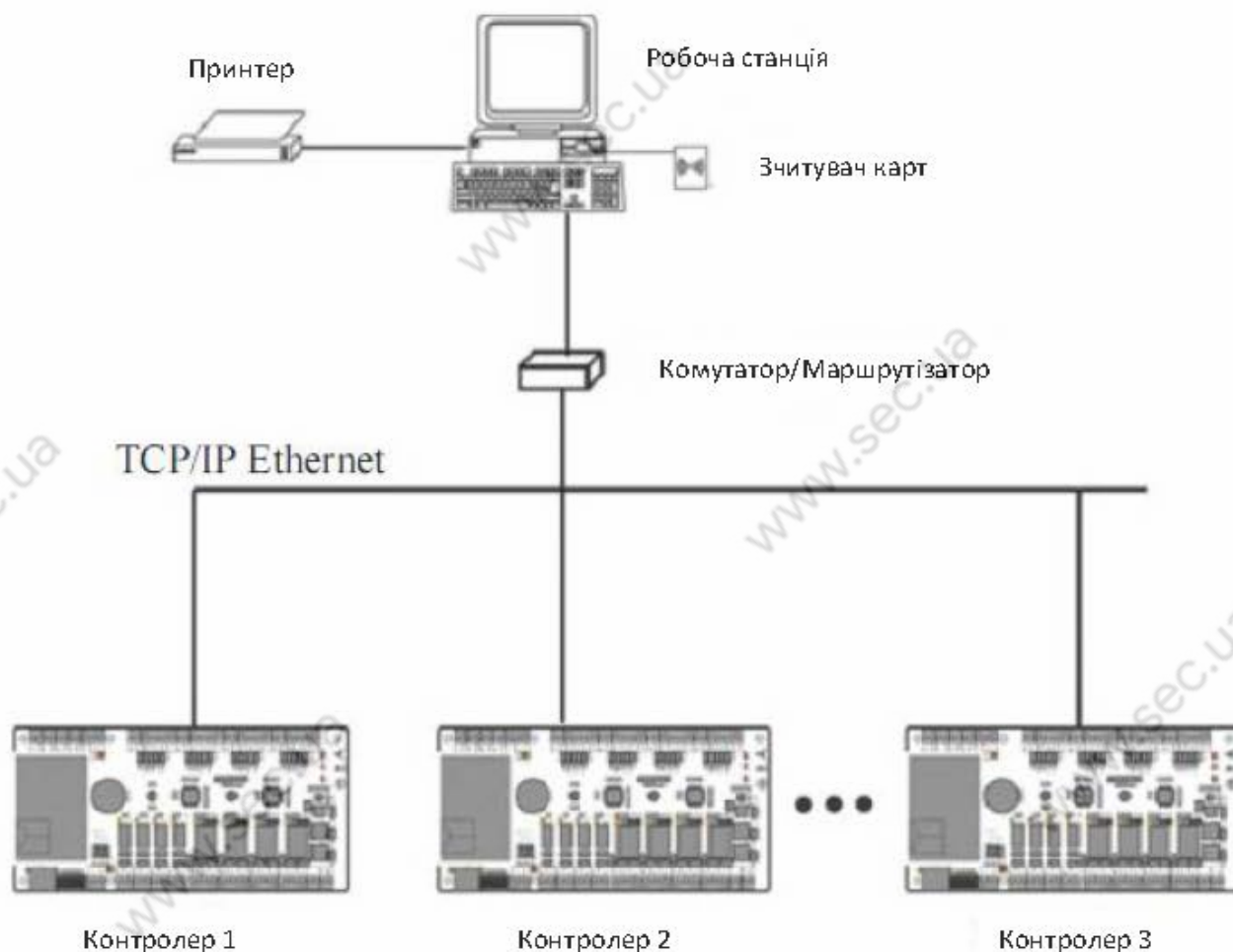
Топологія TCP/IP
