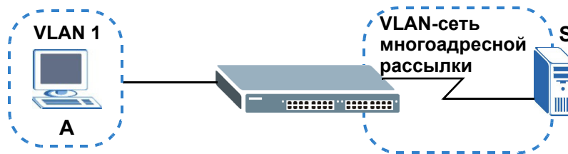
Рисунок 115 Пример с многоадресной рассылкой телевидения посредством MVR
