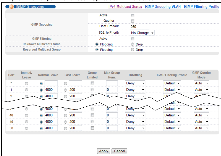
Рисунок 118 Экран Advanced Application > Multicast > IPv4 Multicast > IGMP Snooping
