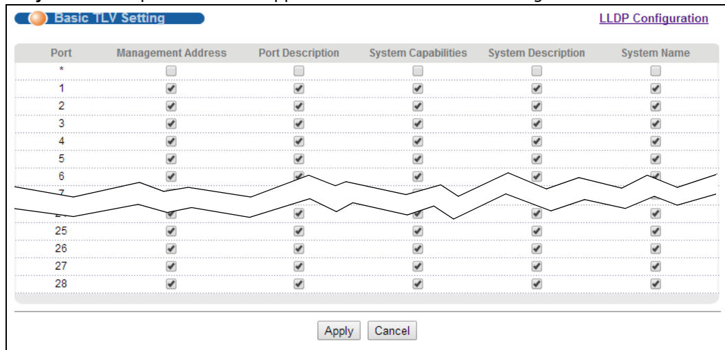
Рисунок 185 Экран Advanced Application &gt; LLDP &gt; LLDP Configuration &gt; Basic TLV Setting
