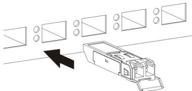
Рисунок 11 Подключение оптоволоконных кабелей
