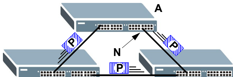
Рисунок 156 Защита от образования петель – петля в сети
