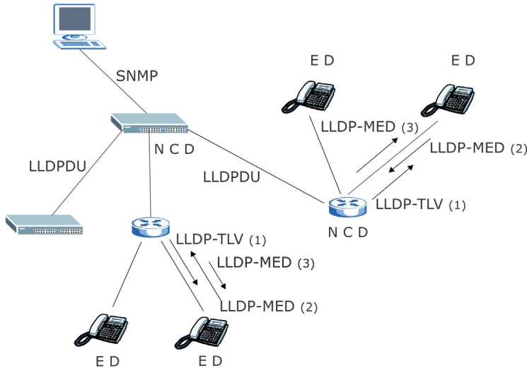
Рисунок 175 Обзор LLDP-MED
