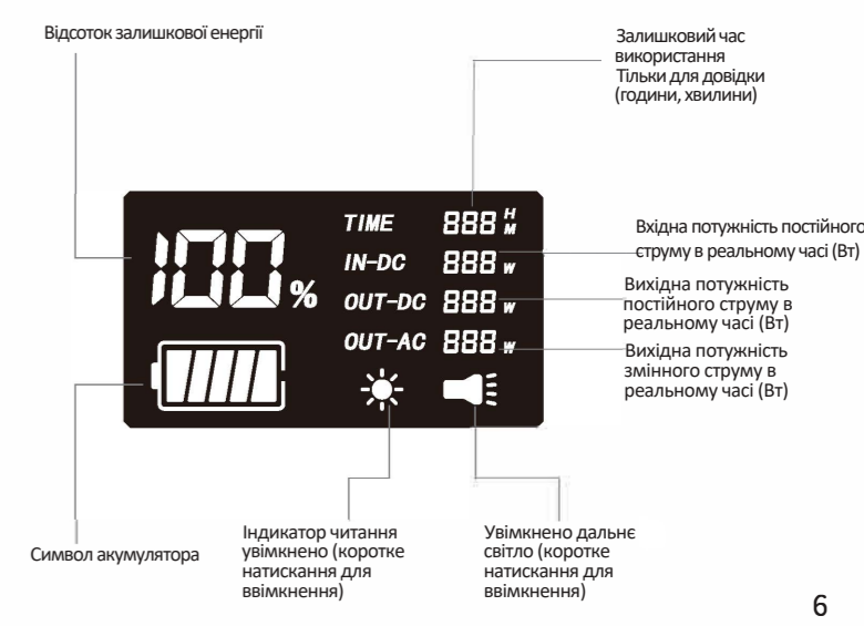
EN700P Дисплей
