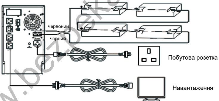
Рис. 3.2.3 Схема підключення батарей до LP UL3500VA
