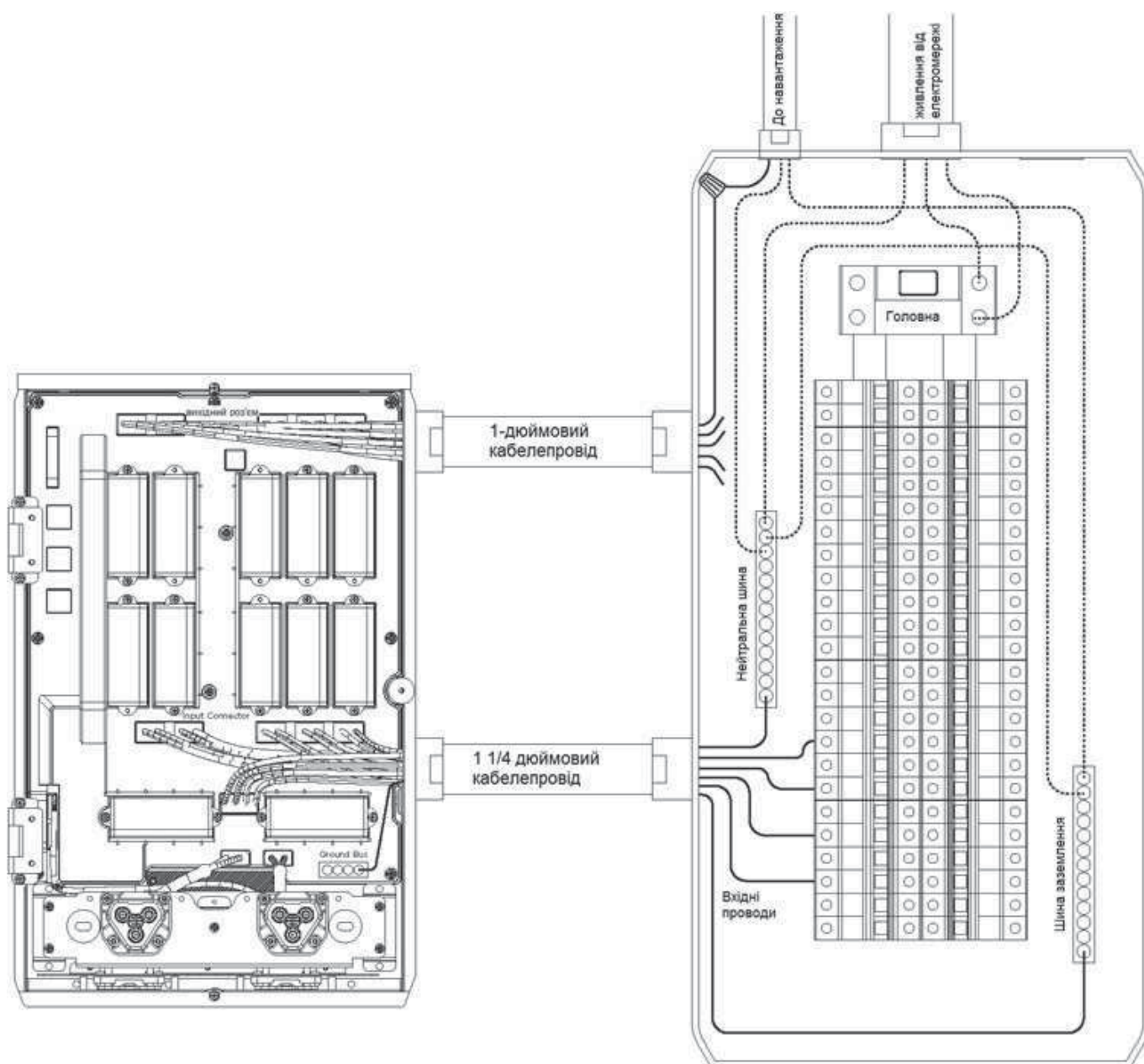
Панель Smart Home
