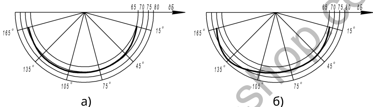
Рисунок 1 – Акустичні діаграми оповіщувачів:
