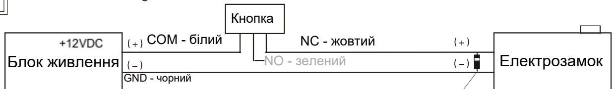
Приклад підключення Fail Safe замка
