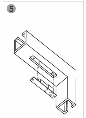
5 Встановіть корпус замка на дверну коробку та протестуйте
