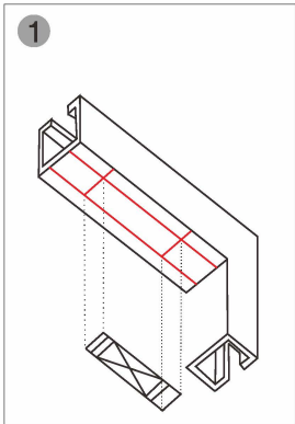
1 Помістіть шаблон корпусу замка на дверну коробку
