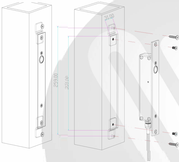
1 Помістіть шаблон корпусу замка на дверну коробку
