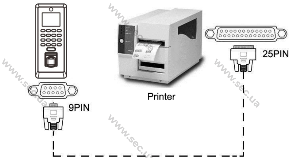
[Схема підключення]
