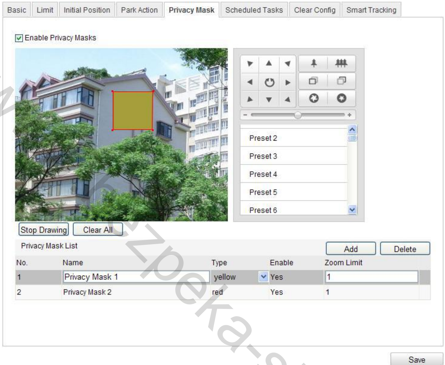
Рисунок 5-9 Область маскирования
