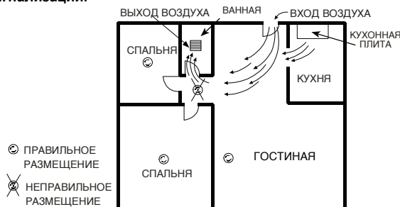
Рис. 10. Рекомендуемые места размещения детекторов для того, чтобы исключить влияние воздушных потоков с частицами продуктов сгорания
