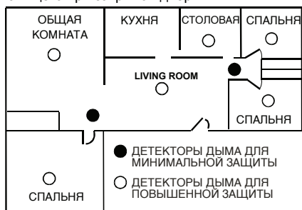
Рис. 6. Расположение детекторов в жилом одноэтажном доме с несколькими спальнями
