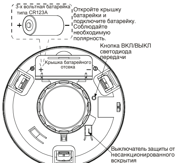
Рис. 3а. Подключение батарейки типа CR123A
